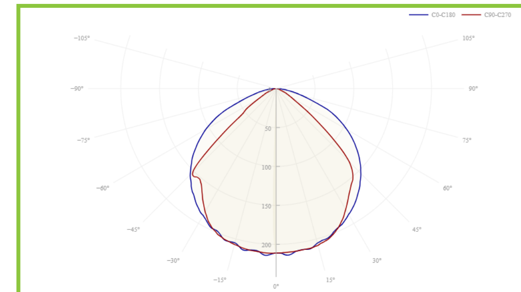
КСС «Д» 96°
