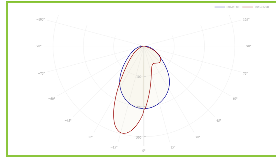
КСС Асимметричный 32°
