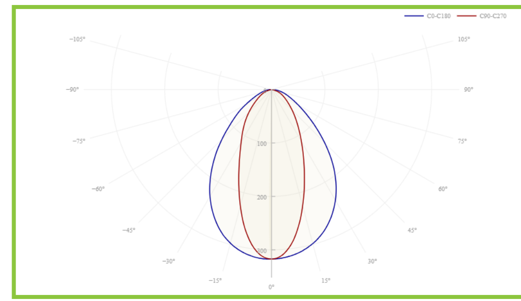
КСС Тип «Д» 85°
