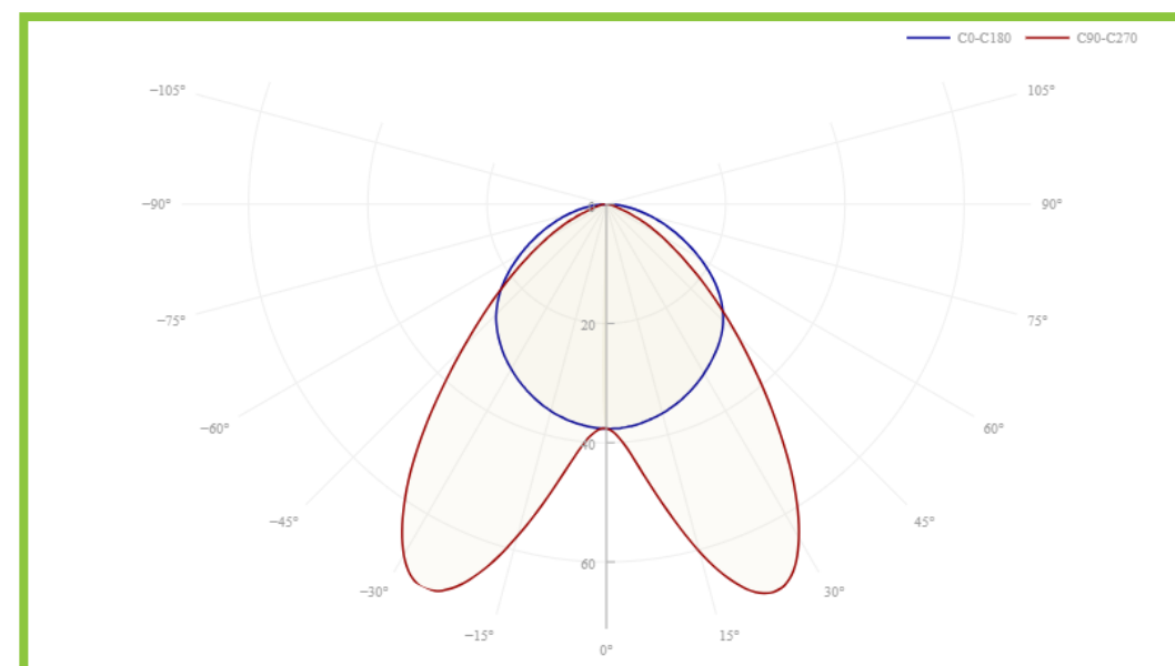
КСС Тип «Л» 96°
