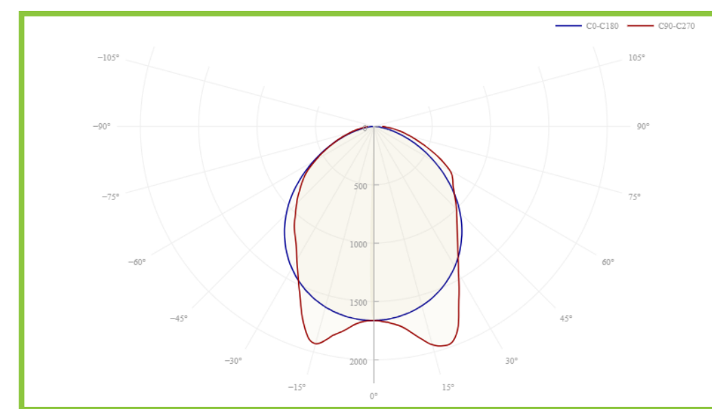
КСС «Л» 92°
