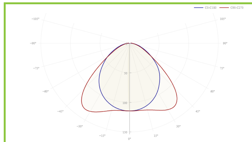
КСС Тип «Л» 108°
