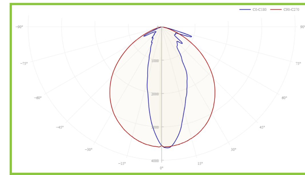
КСС тип «К» 100°
