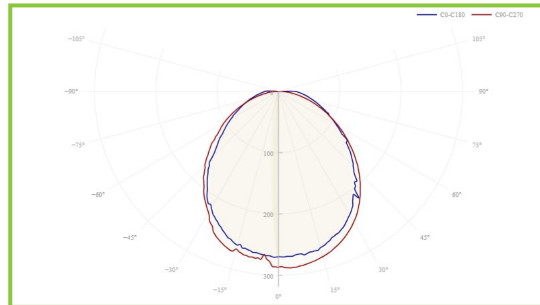
КСС Тип «Д» 110°
